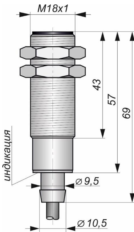
Габаритный чертеж
